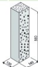
KB palisáda G-B 140-550
