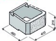
CUP STONE VELKÝ – provedení štípané
