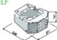
GEOSTONE® - miniSHELF štípaný
