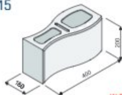
PlayBlok OLYMPIA, barva cihlově-červená
