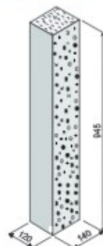
KB palisáda G-B 140-950
