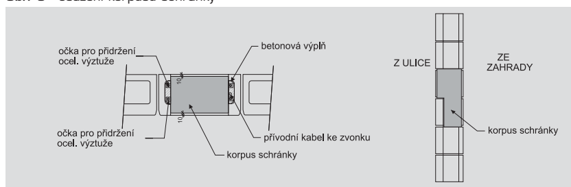
Obr. 3 - osazení korpusu schránky
