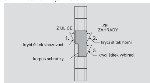
Obr. 4 - osazení krycích štítků
